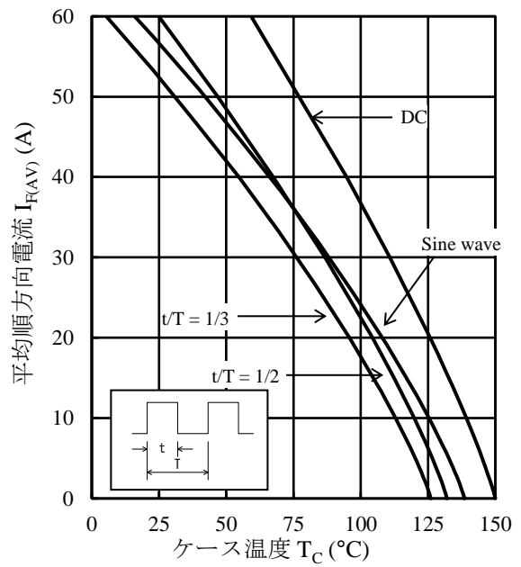
図2 I_{F(AV)} - T_C 特性 ( T_J = 150\text{ }^\circ\text{C} 、 V_R = 600\text{ V} )
