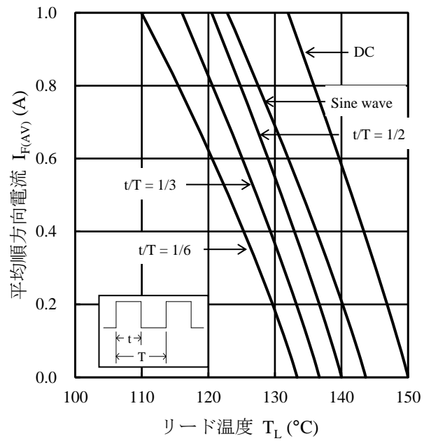
図3 I_{F(AV)} - T_L 特性 (2) ( T_J = 150\text{ }^\circ\text{C} 、 V_R = 1000\text{ V} )
