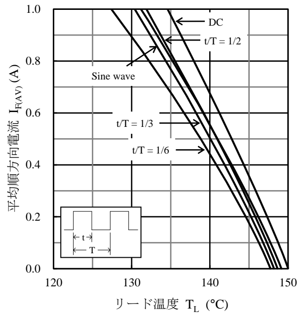
図3 I_{F(AV)} - T_L 特性 (2) ( T_J = 150 °C、 V_R = 800 V)
