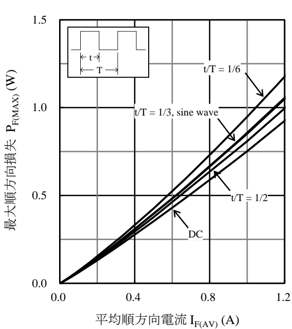
図4 P_{F(MAX)} - I_{F(AV)} 特性 ( T_J = 150^\circ\text{C} )
