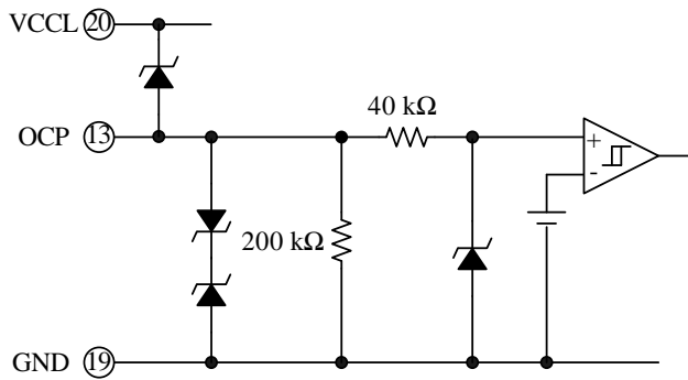
図 9-4 OCP 端子内部回路図
