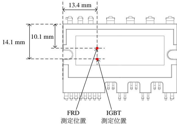
図 5-4 SAM470M30AF1 ケース温度測定位置
