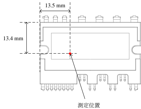
図 2-2 SAM470M50AF1 ケース温度測定位置
