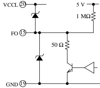
図 9-3 FO 端子内部回路図
