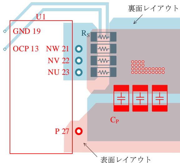
図 15-2 C_P 周辺のレイアウト例（両面基板）
