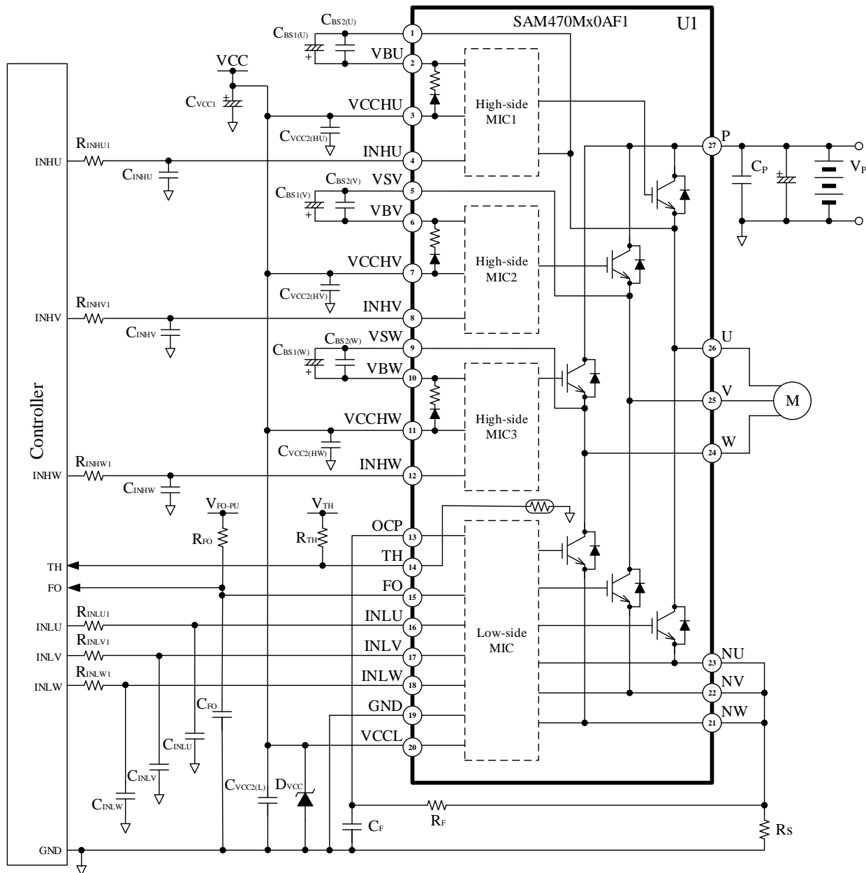
図 11-1 応用回路例
