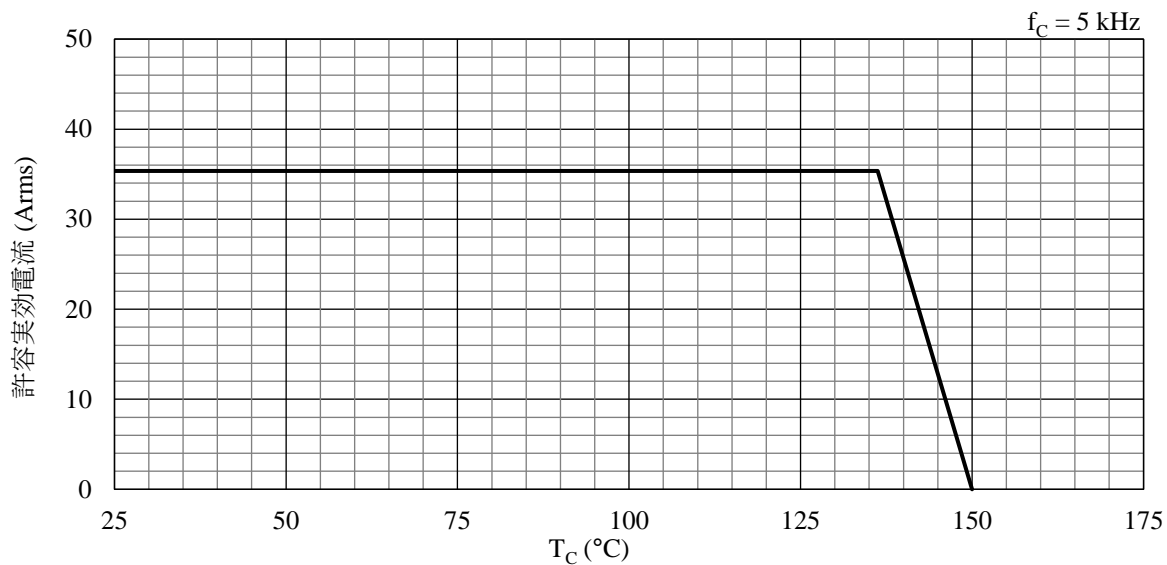
図 17-13 許容電流特性 (f C = 5 kHz)
