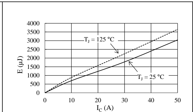
図 17-10 ローサイドスイッチング損失特性
