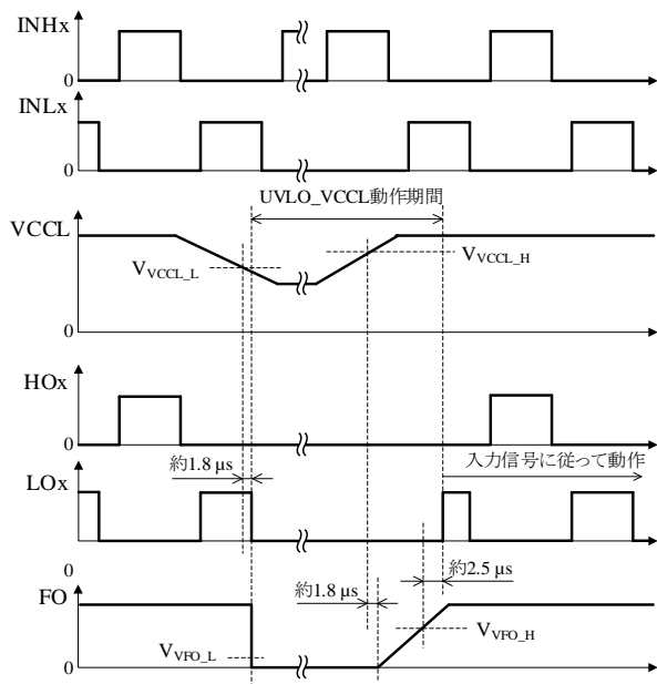
図 14-12 UVLO_VCCL 動作波形
