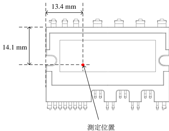
図 2-1 SAM470M30AF1 ケース温度測定位置
