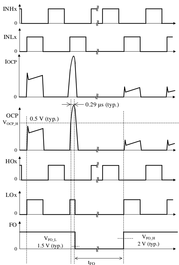
図 14-14 OCP 動作波形
