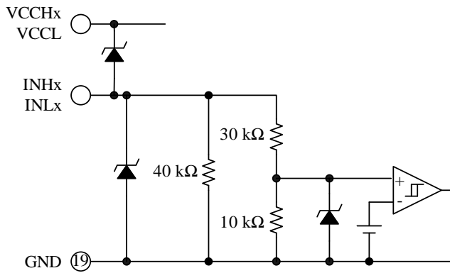
図 9-2 INHx、INLx 端子内部回路図
