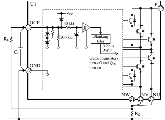
図 14-13 OCP 端子の周辺回路と内部回路
