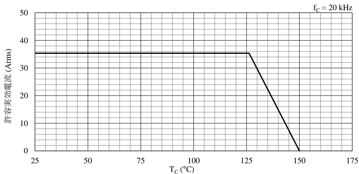
図 17-14 許容電流特性 (f C = 20 kHz)
