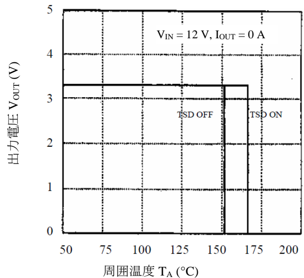
図 13-4 過熱保護特性
