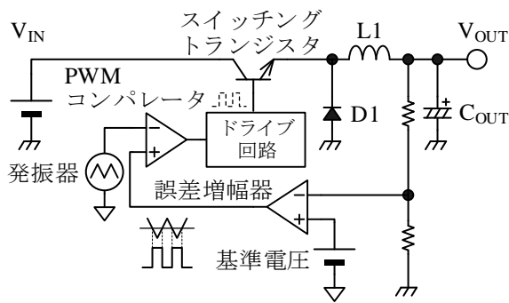
図 10-1 PWM 制御スイッチングレギュレータ基本構成
