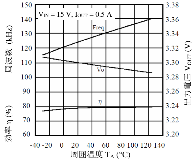
図 13-6 温度特性
