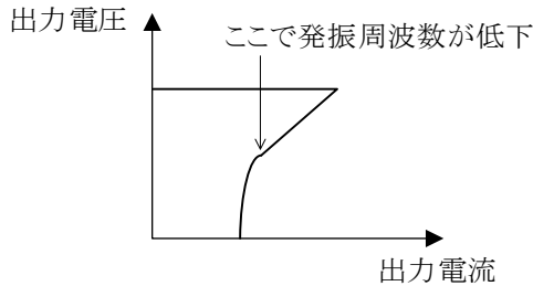
図 10-5 過電流保護特性
