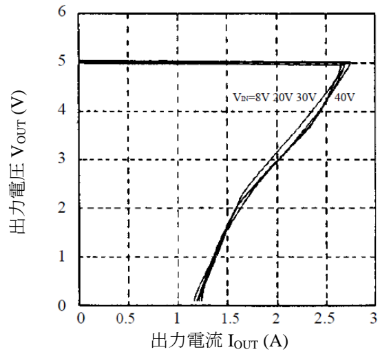
図 13-8 過電流保護特性
