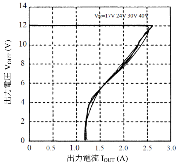
図 13-20 過電流保護特性
