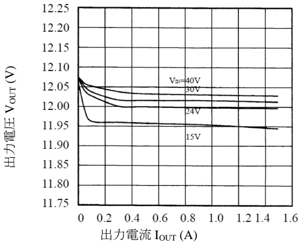
図 13-23 ロードレギュレーション
