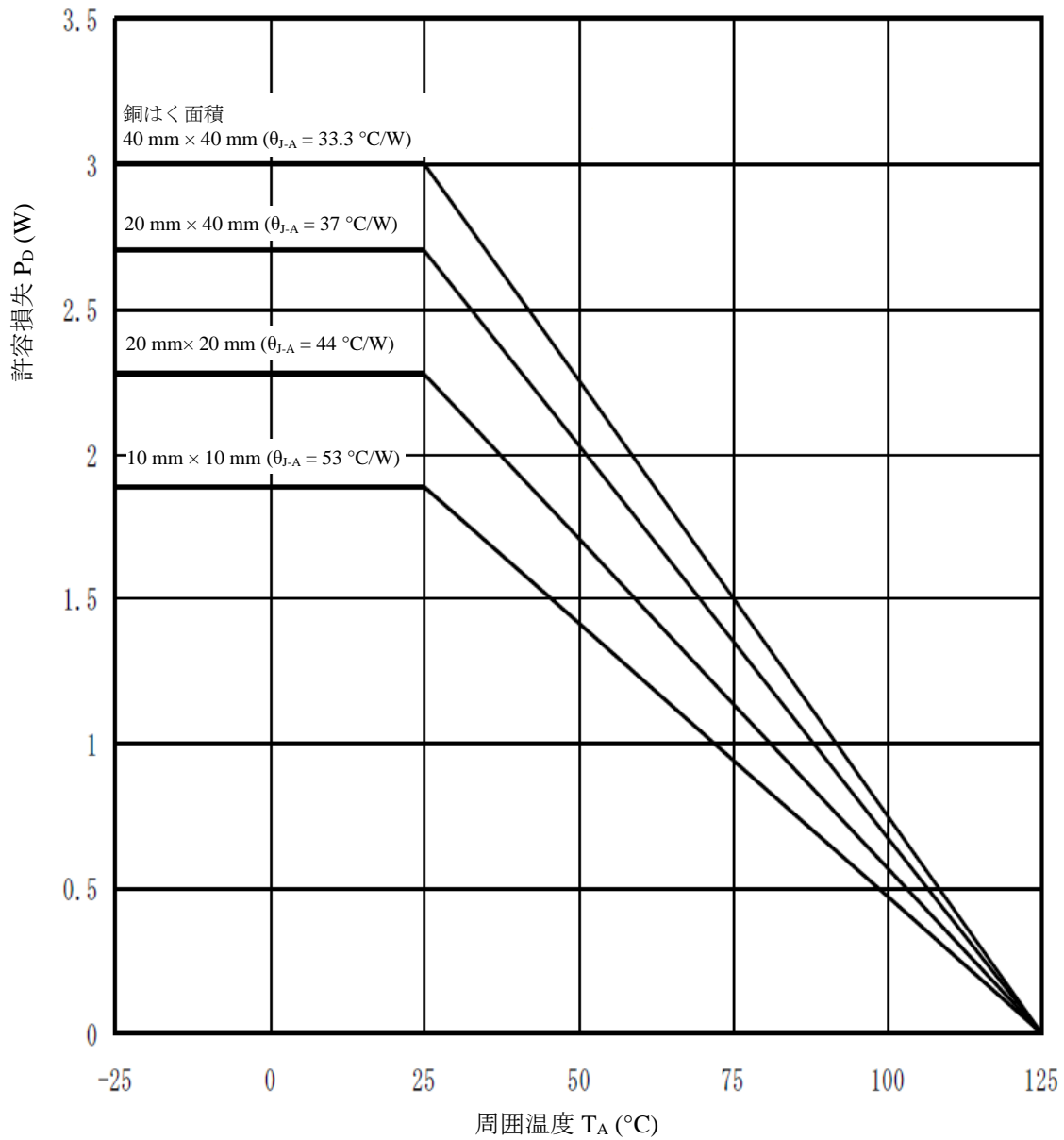
図 13-25 熱減定格
