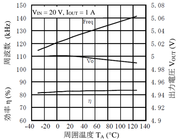
図 13-12 温度特性
