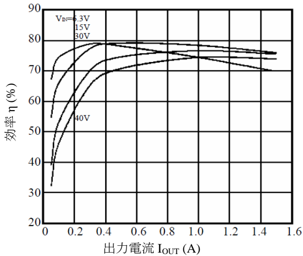
図 13-1 効率
