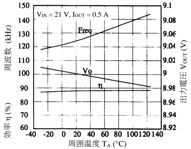
図 13-18 温度特性
