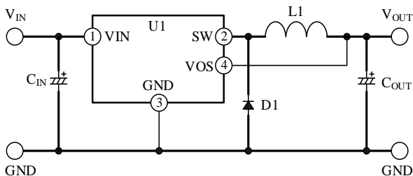
図 11-10 大電流ライン
