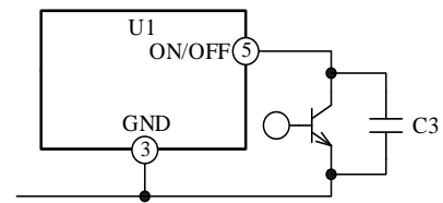
図 10-8 立ち上がり遅延時間の設定
