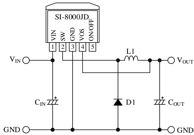
図 7-1 応用回路例
