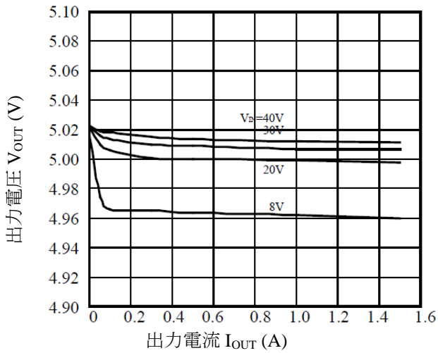
図 13-11 ロードレギュレーション
