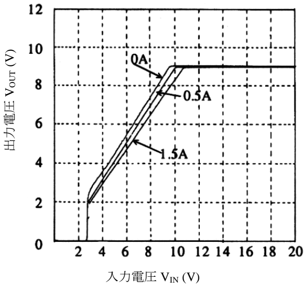
図 13-15 立ち上がり特性
