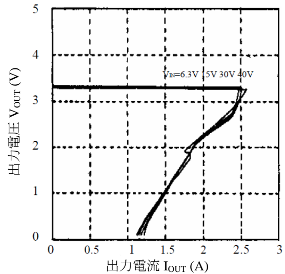
図 13-2 過電流保護特性
