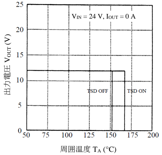
図 13-22 過熱保護特性
