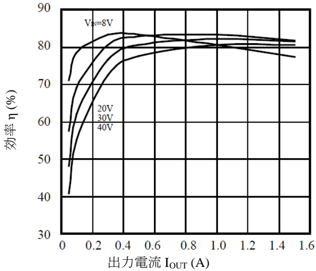
図 13-7 効率
