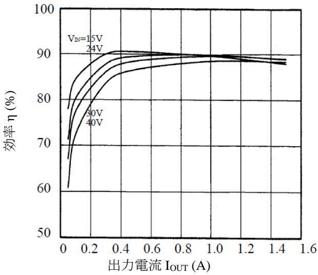
図 13-19 効率
