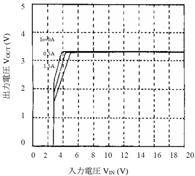
図 13-3 立ち上がり特性
