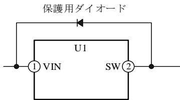
図 11-9 逆バイアス保護用ダイオードの追加
