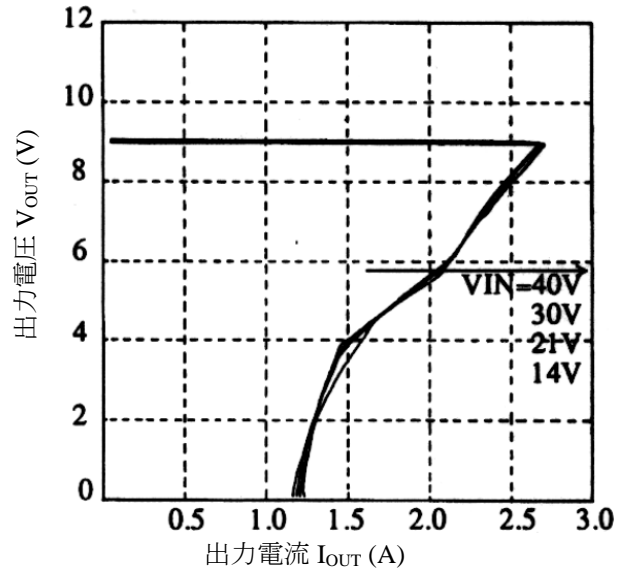
図 13-14 過電流保護特性
