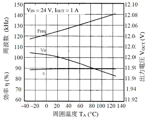
図 13-24 温度特性
