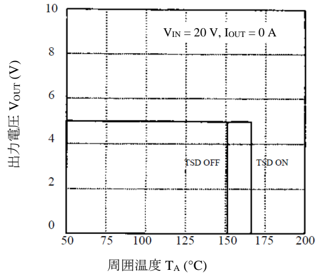
図 13-10 過熱保護特性
