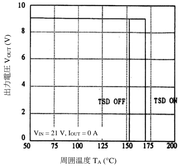
図 13-16 過熱保護特性
