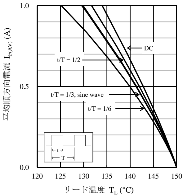
図2 I_{F(AV)} - T_L 代表特性 ( T_J = 150 °C、 V_R = 0 V)
