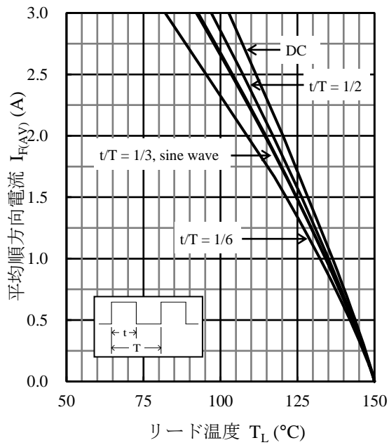
図2 I_{F(AV)} - T_L 特性 ( T_J = 150 °C、 V_R = 0 V)
