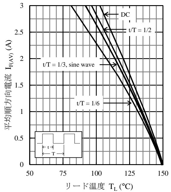
図3 I_{F(AV)} - T_L 特性 ( T_J = 150 °C、 V_R = 200 V)
