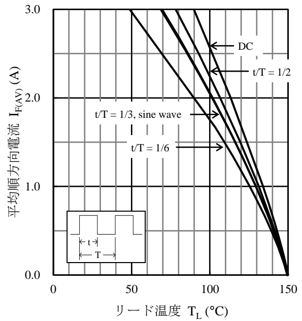
図3 I_{F(AV)} - T_L 特性 ( T_J = 150 °C、 V_R = 400 V)
