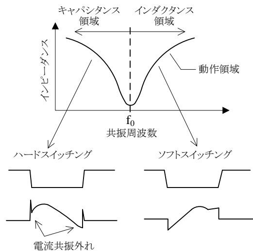
図 8-29 共振電源の動作領域
