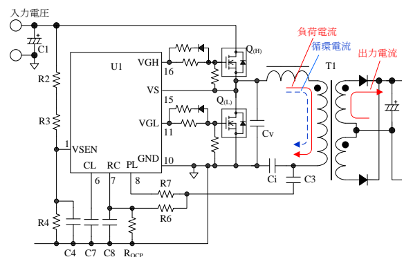
図 8-38 PL、CL 端子周辺回路
