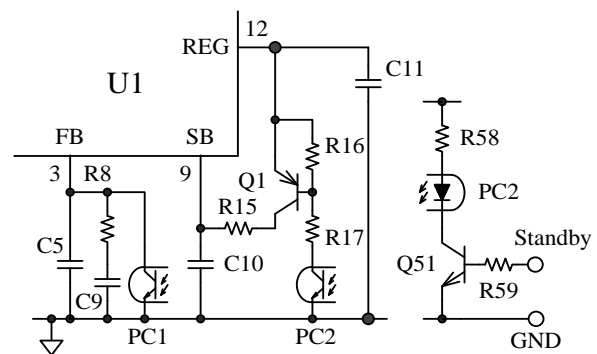
図 8-20 スタンバイ切り替え回路
