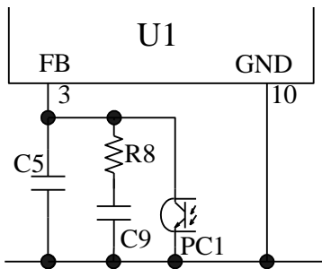
図 8-18 FB 端子周辺回路
