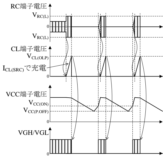
図 8-37 OLP 動作波形
