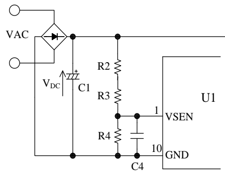
図 8-28 VSEN 端子周辺回路
