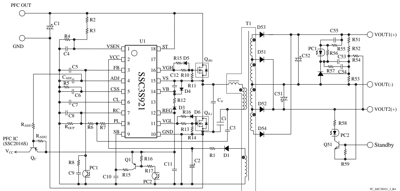
図 5-1 応用回路例
