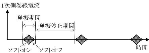
図 8-19 スタンバイ動作波形
