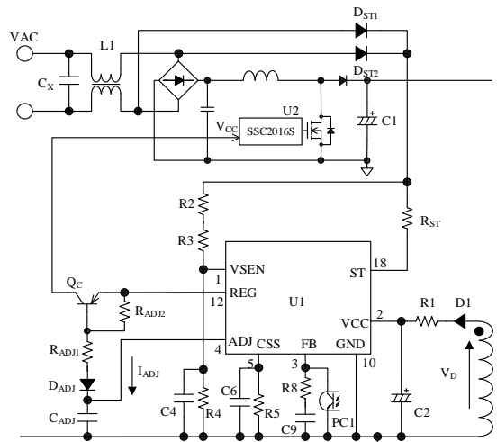
図 8-11 VCC 端子周辺回路
