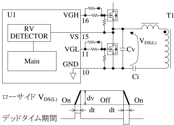
図 8-26 VS 端子とデッドタイム期間
