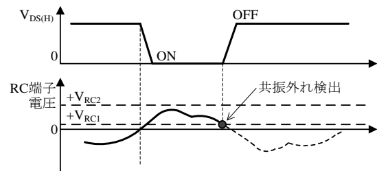
図 8-31 ハイサイド側電流共振外れ検出 (軽負荷時)
