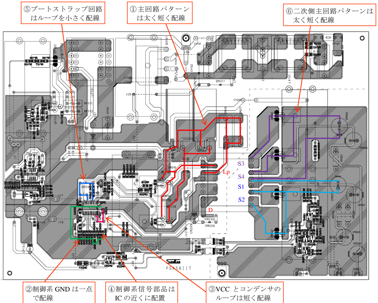
図 10-1 パターンレイアウト例
