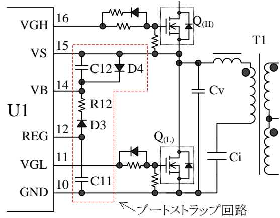
図 8-17 ブートストラップ回路
