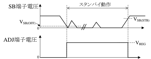
図 8-23 PFC ON/OFF 機能
