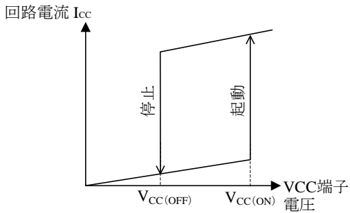
図 8-13 VCC 端子電圧と回路電流 I_{CC}
