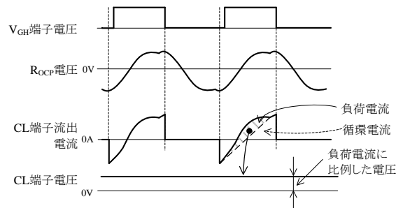
図 8-39 CL 端子動作波形
