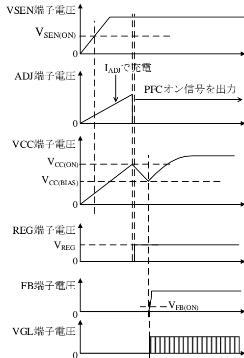
図 8-12 PFC オン/オフ信号を使用する場合の起動動作
