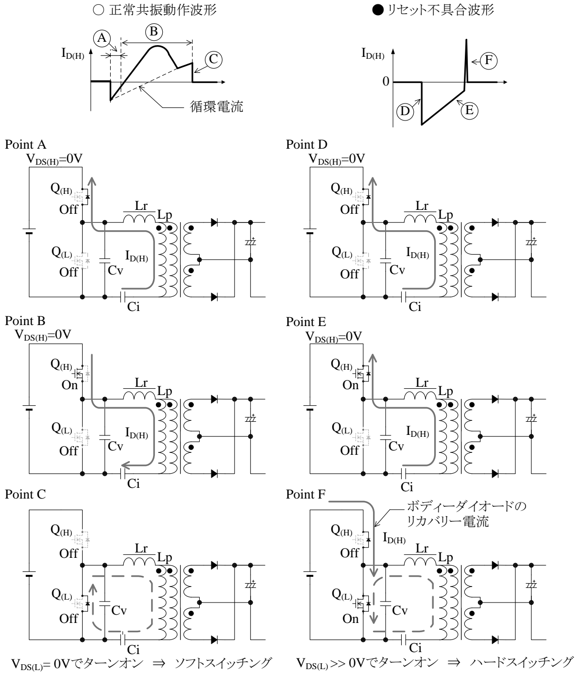
図 8-35 正常共振動作とリセット不具合のハイサイド側の動作とドレイン電流波形例
