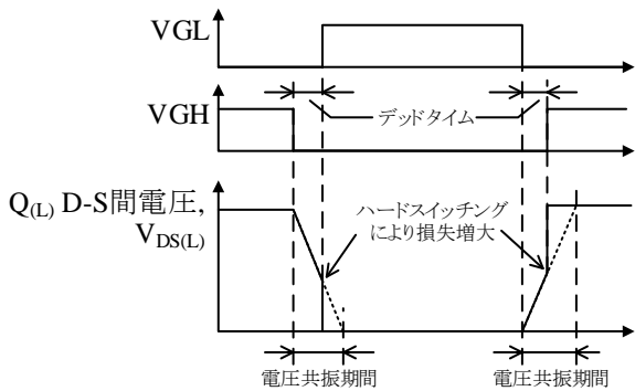
図 8-25 ZVS 不具合波形
