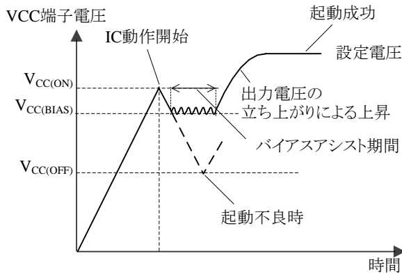
図 8-14 起動時の VCC 端子電圧
