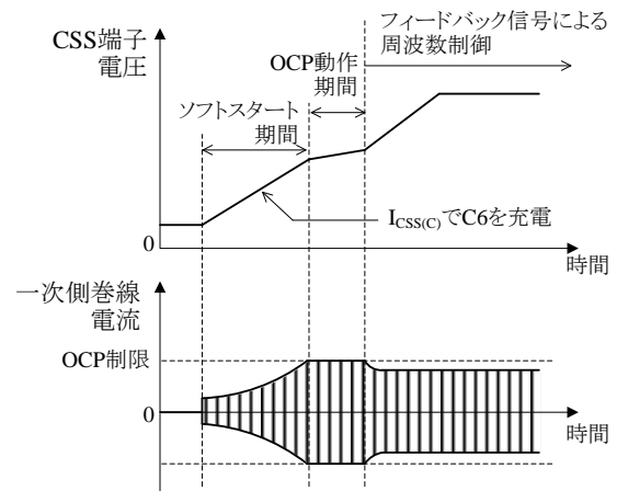
図 8-15 ソフトスタート動作
