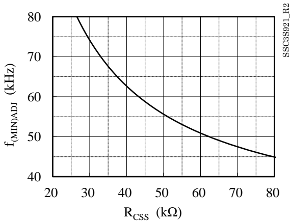
図 8-16 R5 ( R_{CSS} ) と f_{(MIN)ADJ} 特性
