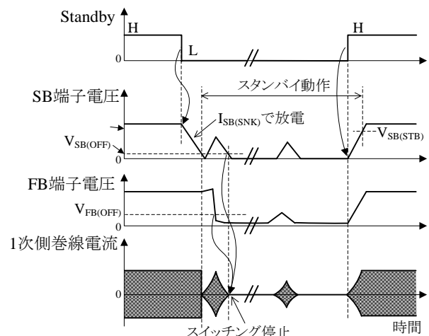
図 8-21 スタンバイ切り替え動作波形
