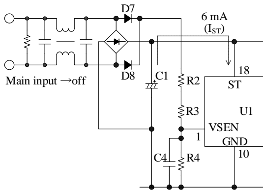
図 8-33 入力コンデンサの残留電圧放電
