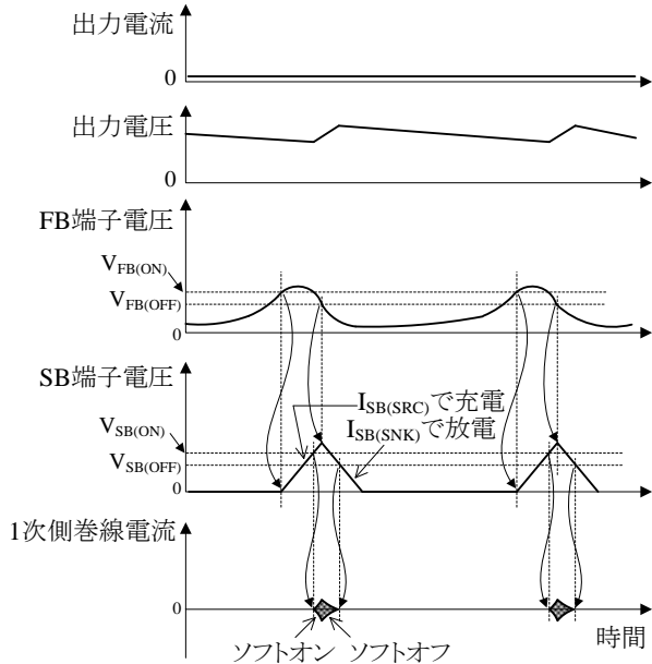
図 8-22 バースト発振動作
