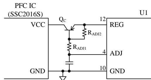
図 8-24 ADJ 端子の信号で PFC IC を停止する場合の回路例 ( V_{CC(ON\_PFC)} < V_{REG} )
