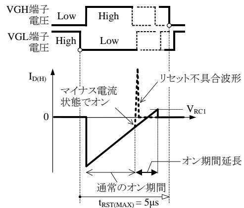
図 8-34 ハイサイドオン期間のリセット検出機能動作例
