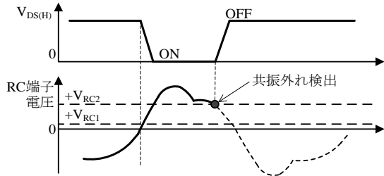
図 8-32 ハイサイド側電流共振外れ検出 (重負荷時)
