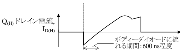
図 8-27 ZCS 確認箇所
