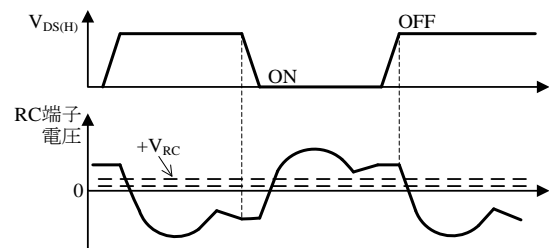
図 8-30 インダクタンス領域の RC 端子の波形
