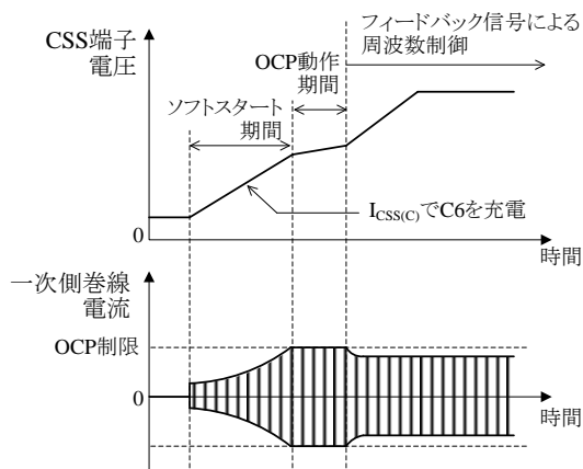
図 8-15 ソフトスタート動作
