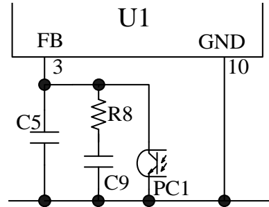
図 8-18 FB 端子周辺回路
