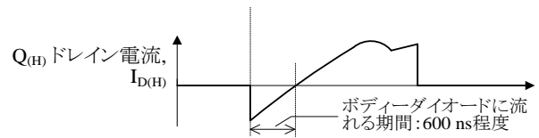
図 8-25 ZCS 確認箇所
