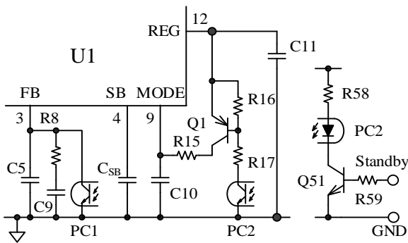
図 8-20 スタンバイ切り替え回路
