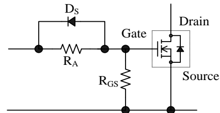
図 9-1 パワーMOSFET ゲート周辺回路
