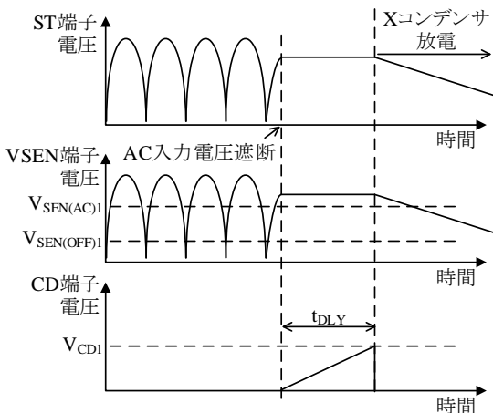
図 8-32 X コンデンサ放電機能動作波形
