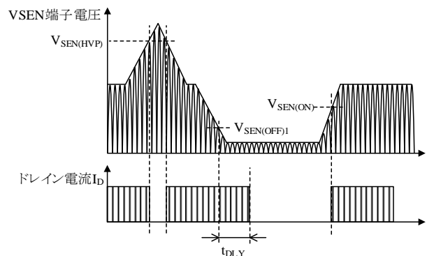
図 8-37 入力電圧検出機能動作波形
