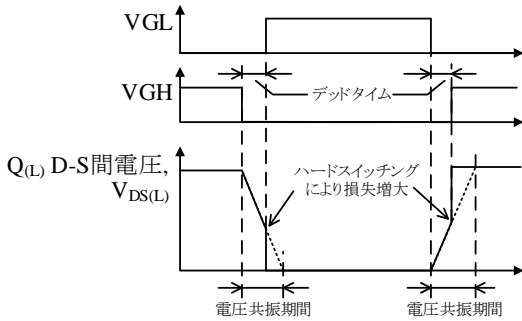
図 8-23 ZVS 不具合波形
