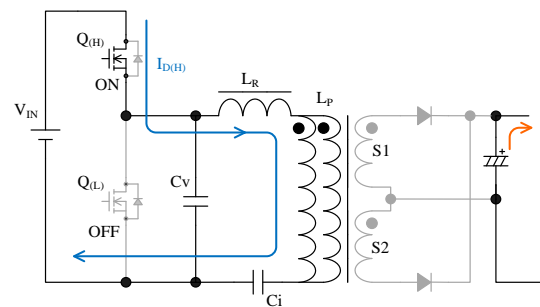
図 8-6 期間 B の動作
