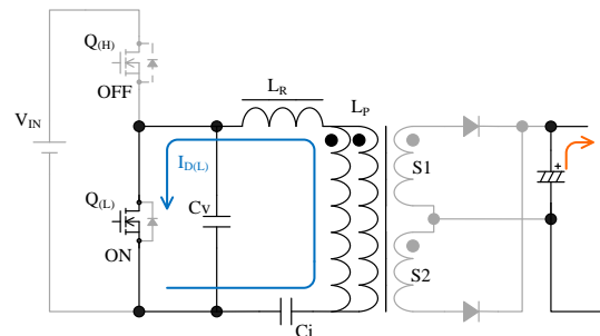
図 8-9 期間 E の動作
