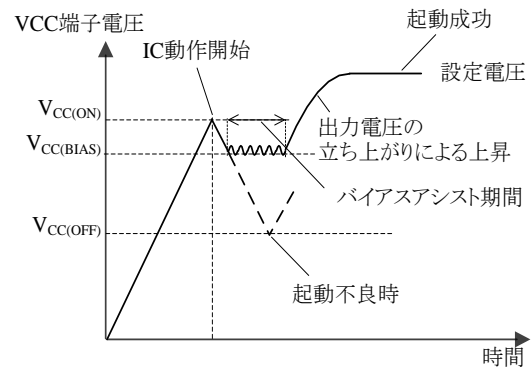
図 8-14 起動時の V_{CC} 端子電圧
