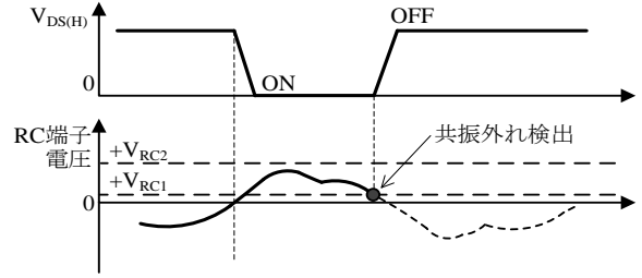
図 8-28 ハイサイド側電流共振外れ検出 (軽負荷時)
