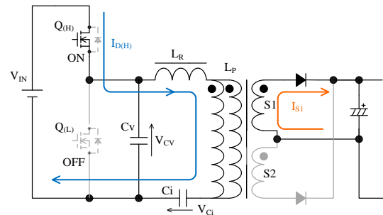
図 8-5 期間 A の動作
