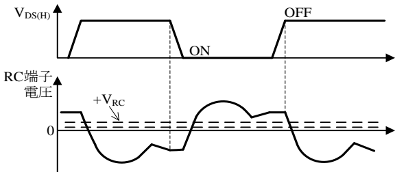
図 8-27 インダクタンス領域の RC 端子の波形
