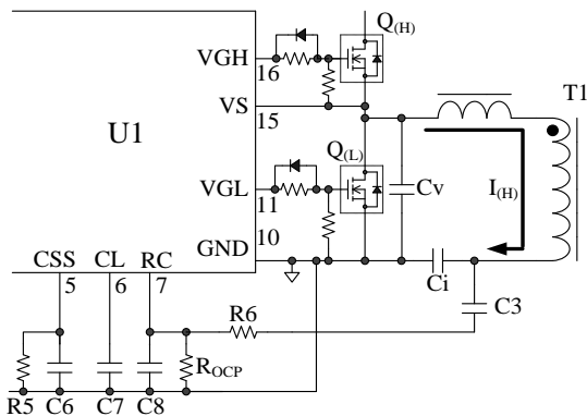
図 8-38 RC 端子周辺回路
