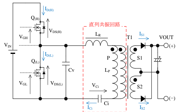
図 8-3 電流共振電源回路図
