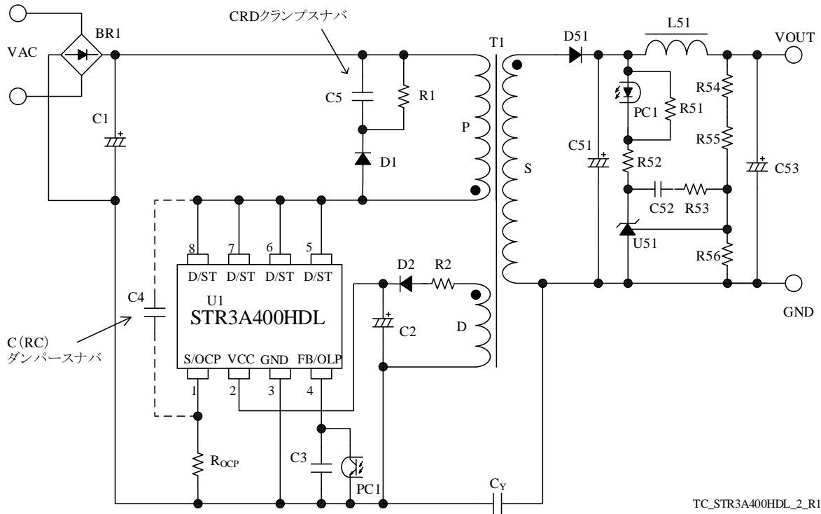
図 7-1 応用回路例
