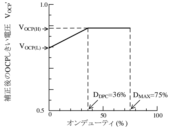
図 10-14 オンデューティと補正後の V_{OCP}
