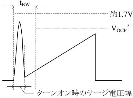
図 10-12 S/OCP 端子電圧波形
