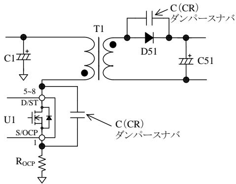
図 10-13 ダンパースナバ
