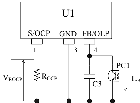
図 10-5 FB/OLP 端子周辺回路
