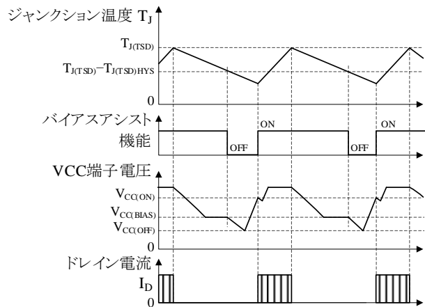
図 10-18 TSD 動作波形
